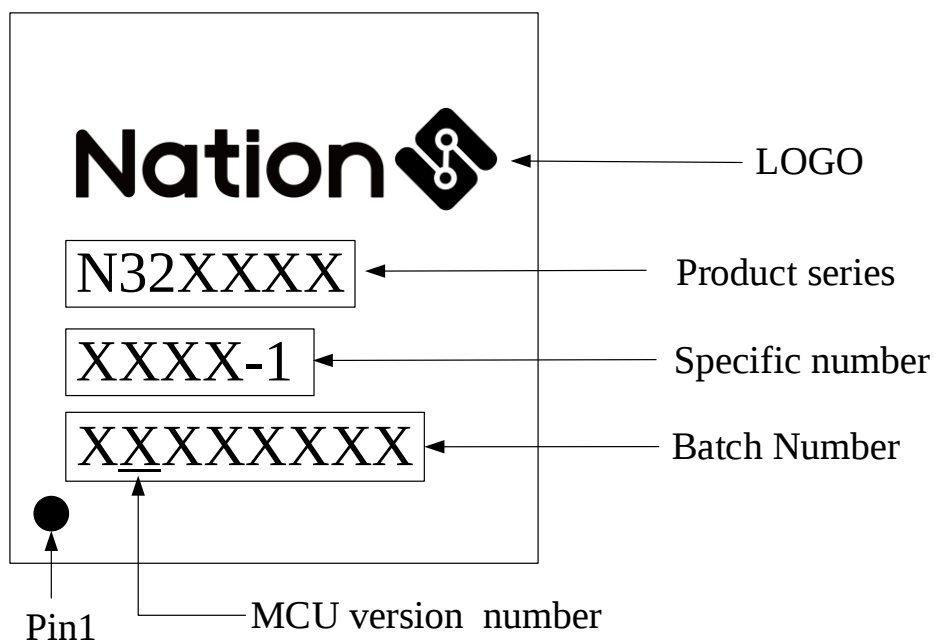
图 5-14 QFN32(4mm x 4mm)丝印说明图
