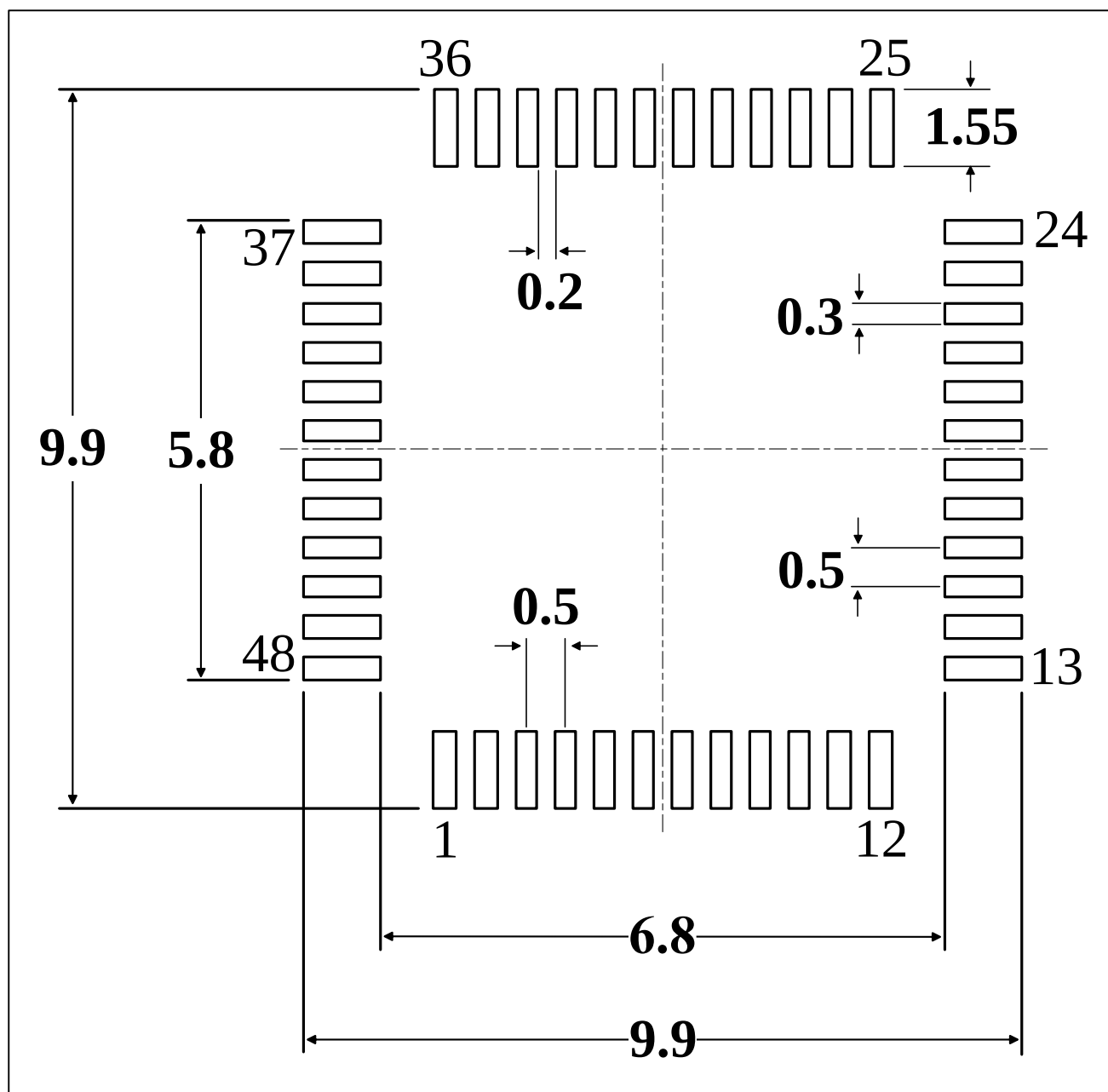
图 5-2 LQFP48 封装焊盘建议 (1)
