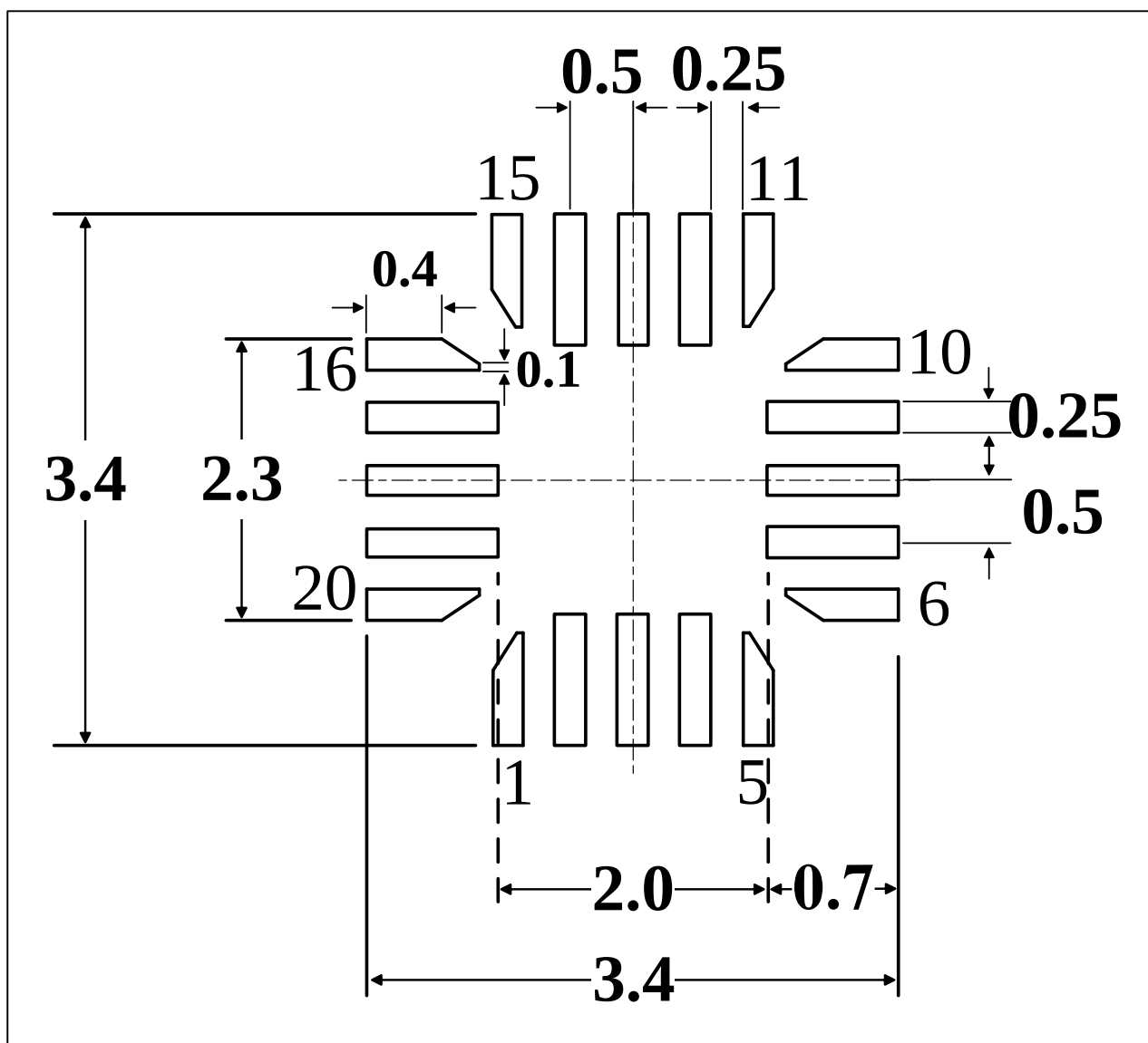
图 5-10 UFQFPN20 封装焊盘建议 (1)
