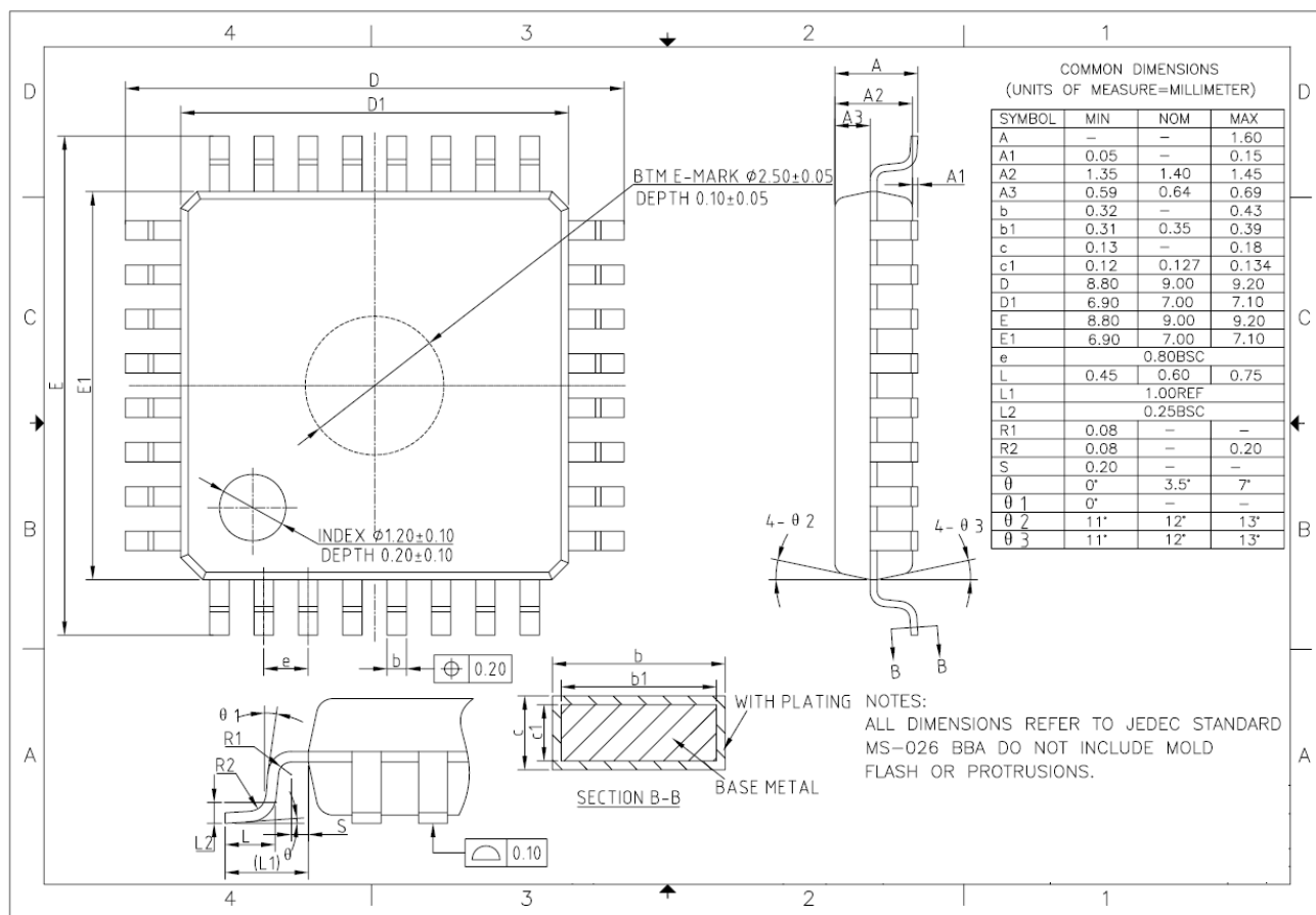
图 5-3 LQFP32 封装尺寸
