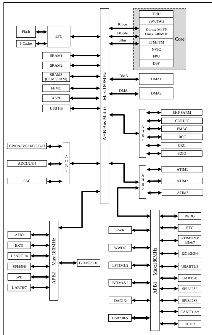
图 1-1 N32H480 系列框图
