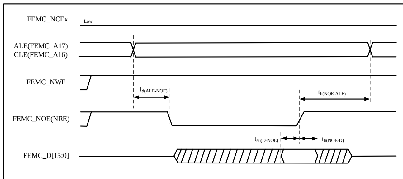
图 4-29 NAND控制器读操作波形
