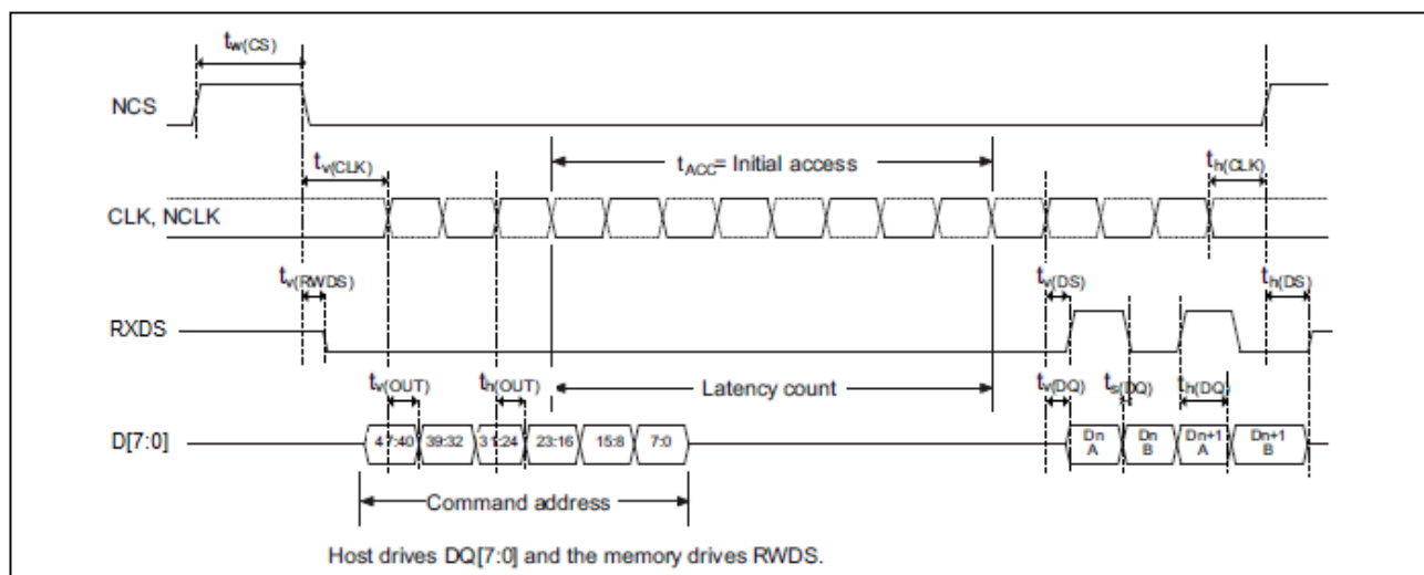
图 4-20 xSPI在RXDS模式下的时序
