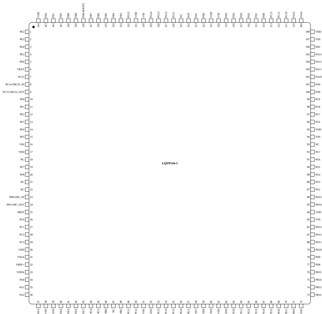
图 3-4 LQFP144-1引脚分布
