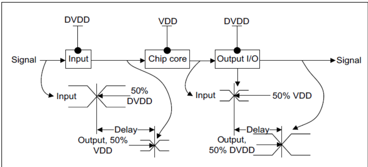
图 4-10 传输延迟
