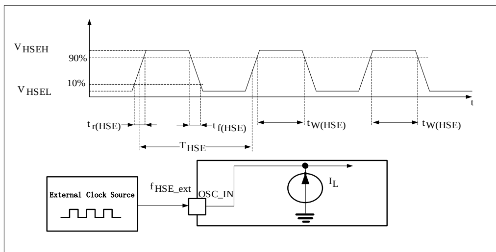
图 4-5 外部高速时钟源的交流时序图
