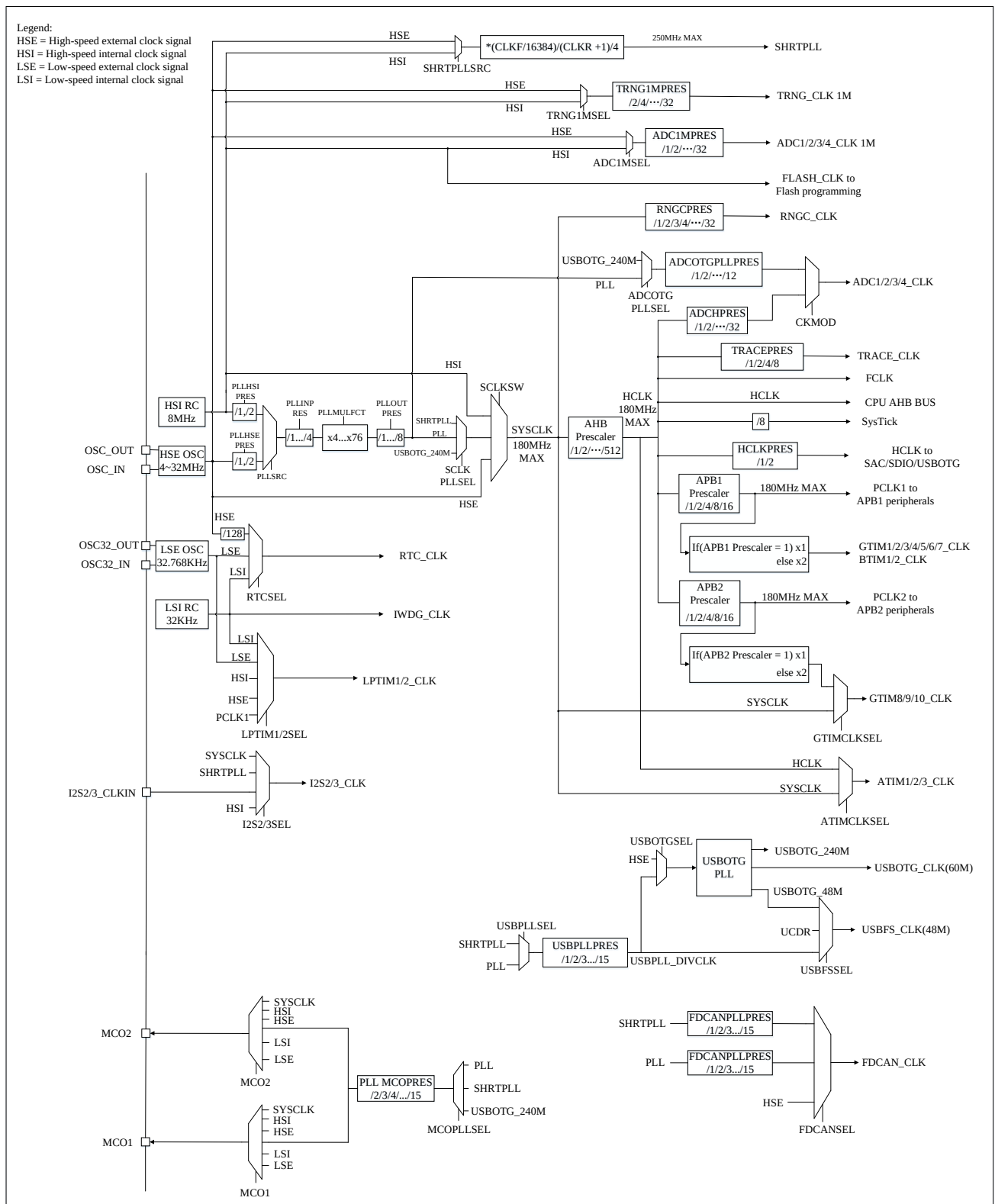
图 2-2 时钟树
