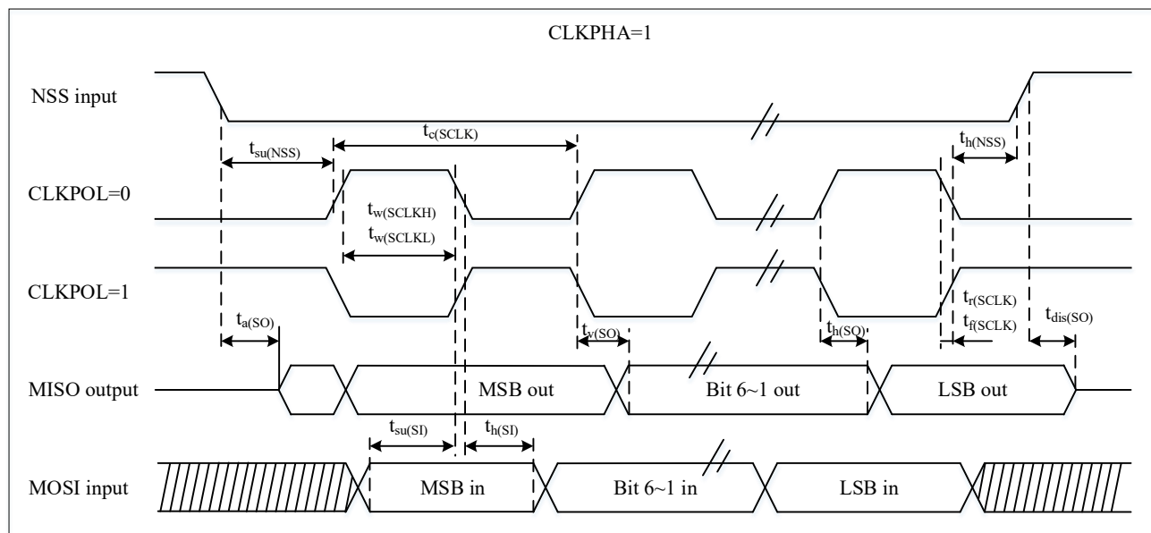
图 4-16 SPI 时序图 — 从模式和 CLKPHA=1 (1)
