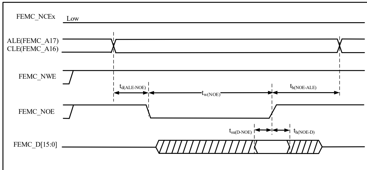
图 4-33 NAND 控制器读操作波形
