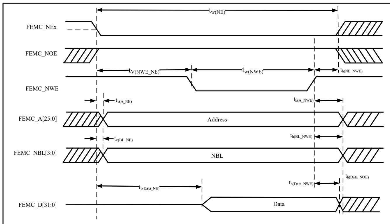
图 4-26 异步非总线复用的 SRAM/PSRAM/NOR 写操作波形
