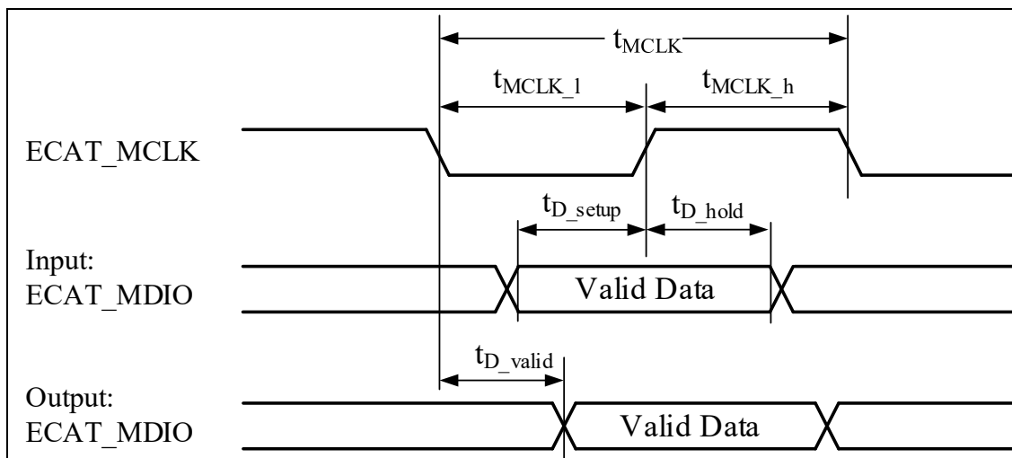
图 4-41 ESC MI (MCLK, MDIO) 时序图
