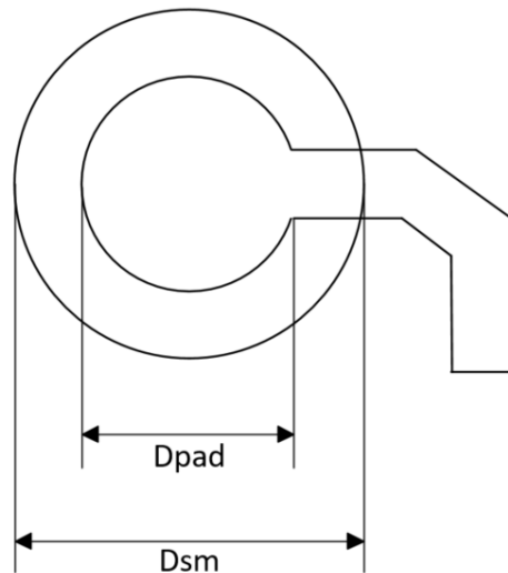
图 5-4 BGA176+25 封装焊盘建议
