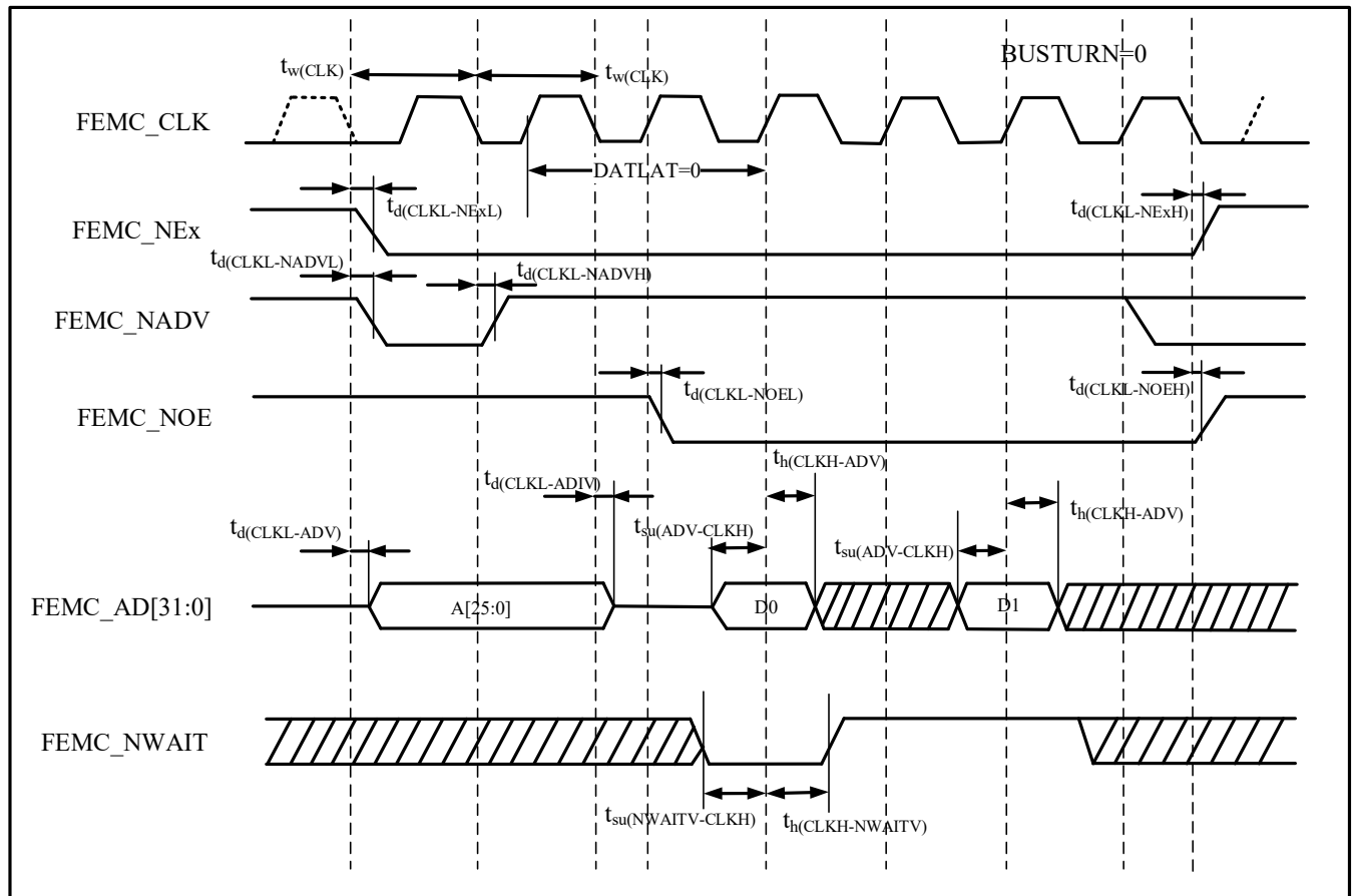
图 4-31 同步复用 NOR/PSRAM 读时序
