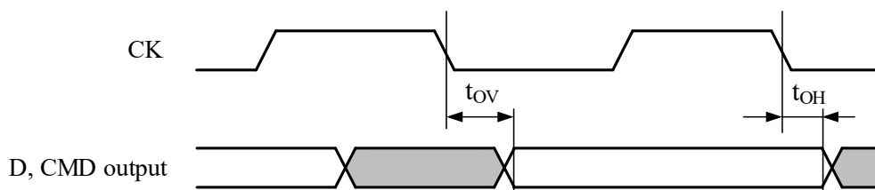
图 4-37 SDMMC DDR 模式
