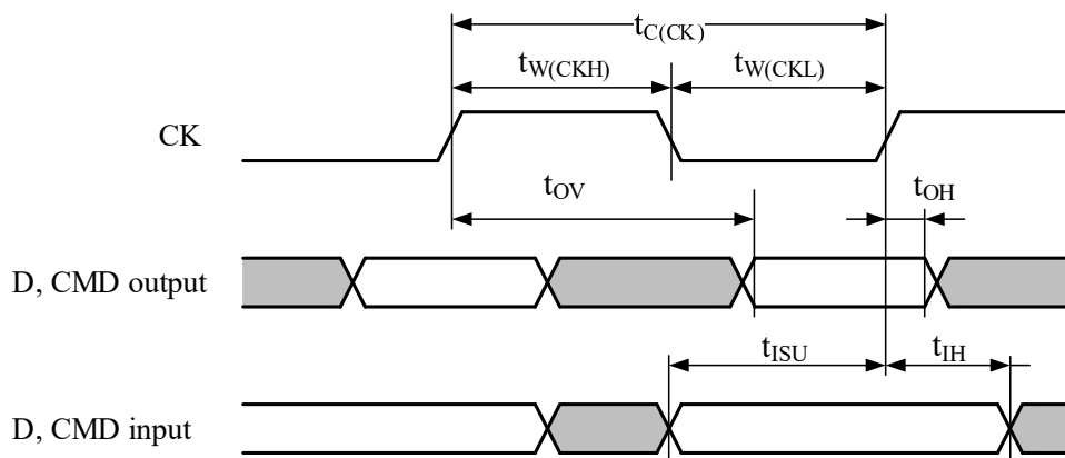
图 4-36 SD 默认模式
