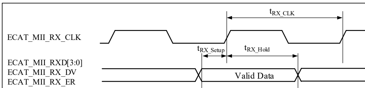
图 4-43 ESC MII RX 信号时序图
