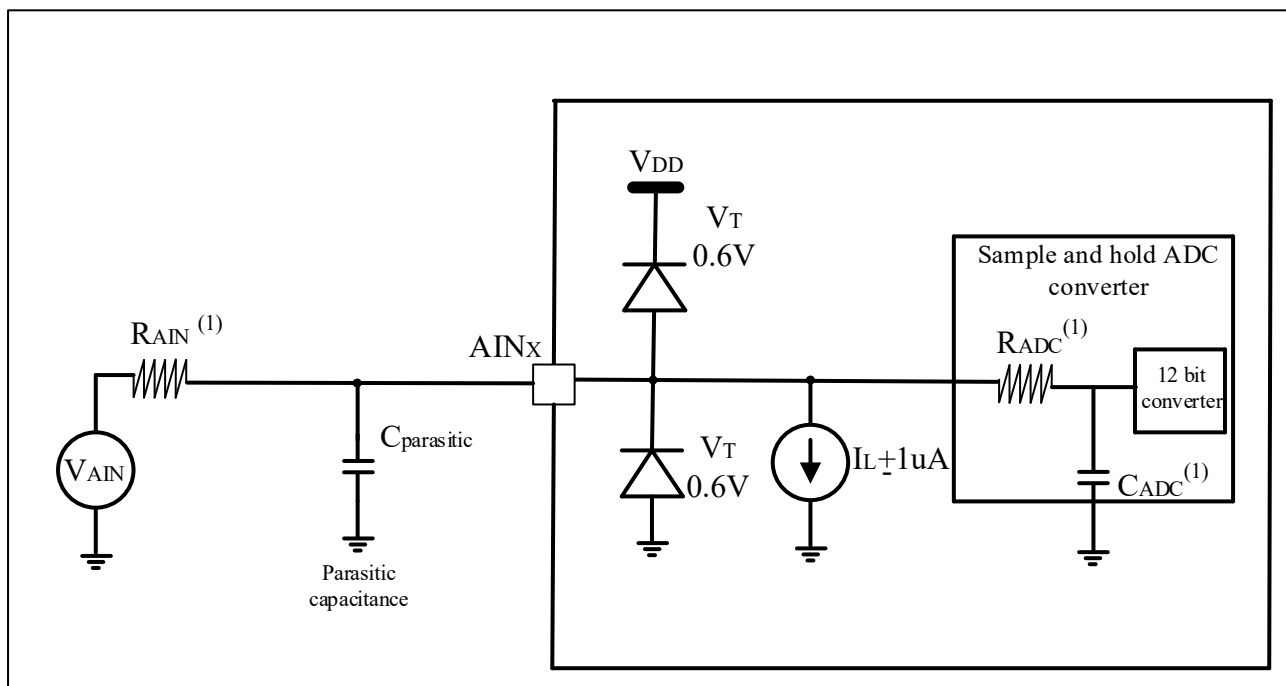
图 4-50 使用 ADC 典型的连接图
