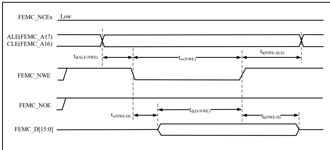
图 4-34 NAND 控制器写操作波形
