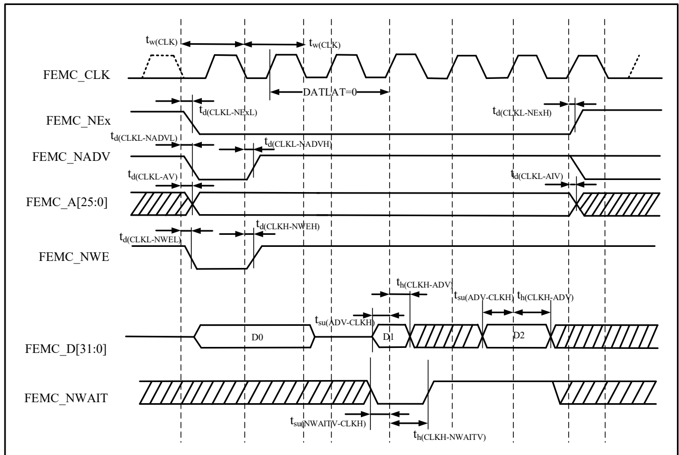
图 4-30 同步非复用 PSRAM 写时序
