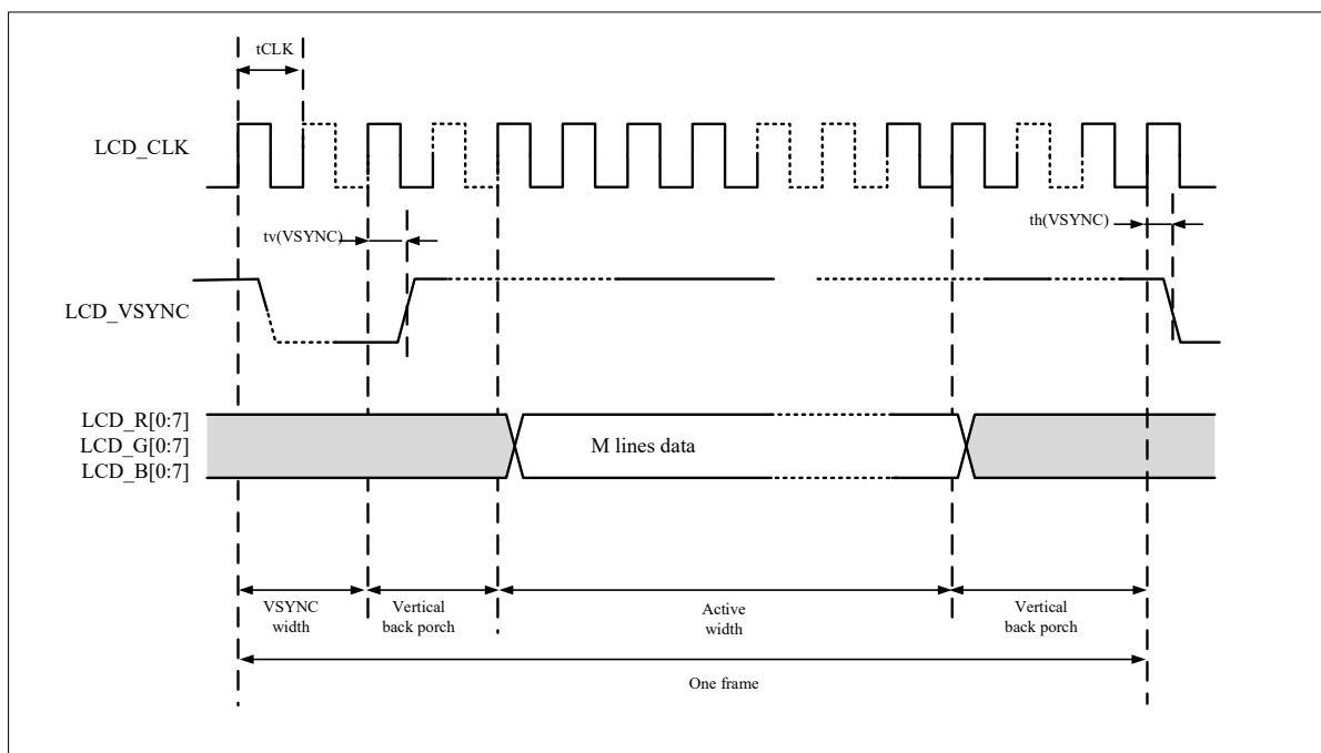
图 4-47 LCDC 垂直时序框图
