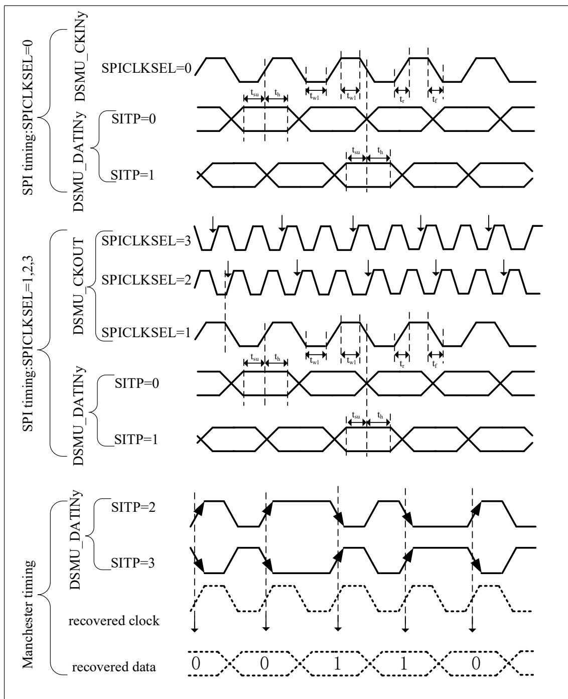
图 4-48 DSMU 通道收发器时序图
