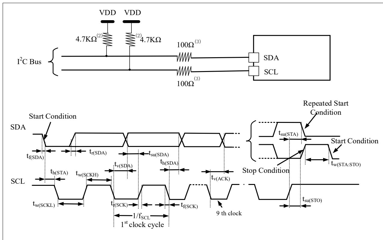
图 4-14 I 2 C 总线交流波形和测量电路 (1)
