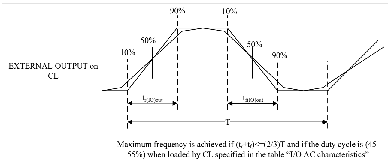
图 4-11 输入输出交流特性定义
