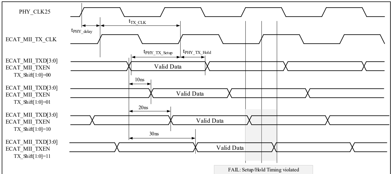
图 4-42 ESC MII TX 信号时序图
