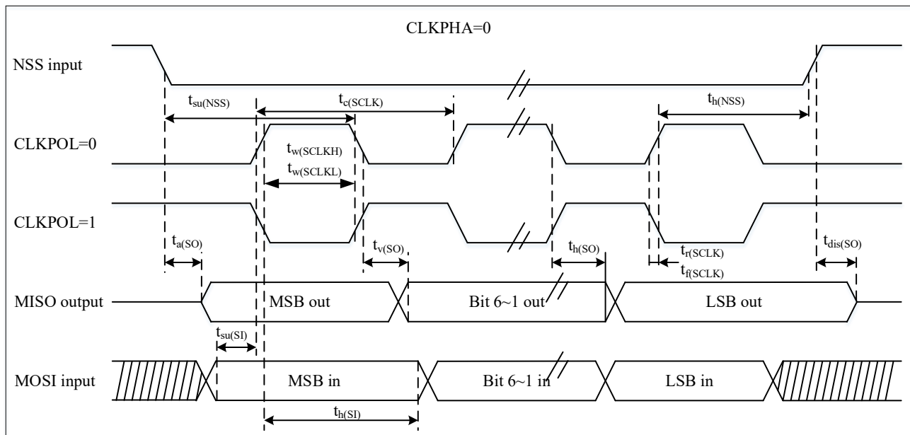
图 4-15 SPI 时序图 – 从模式和 CLKPHA=0
