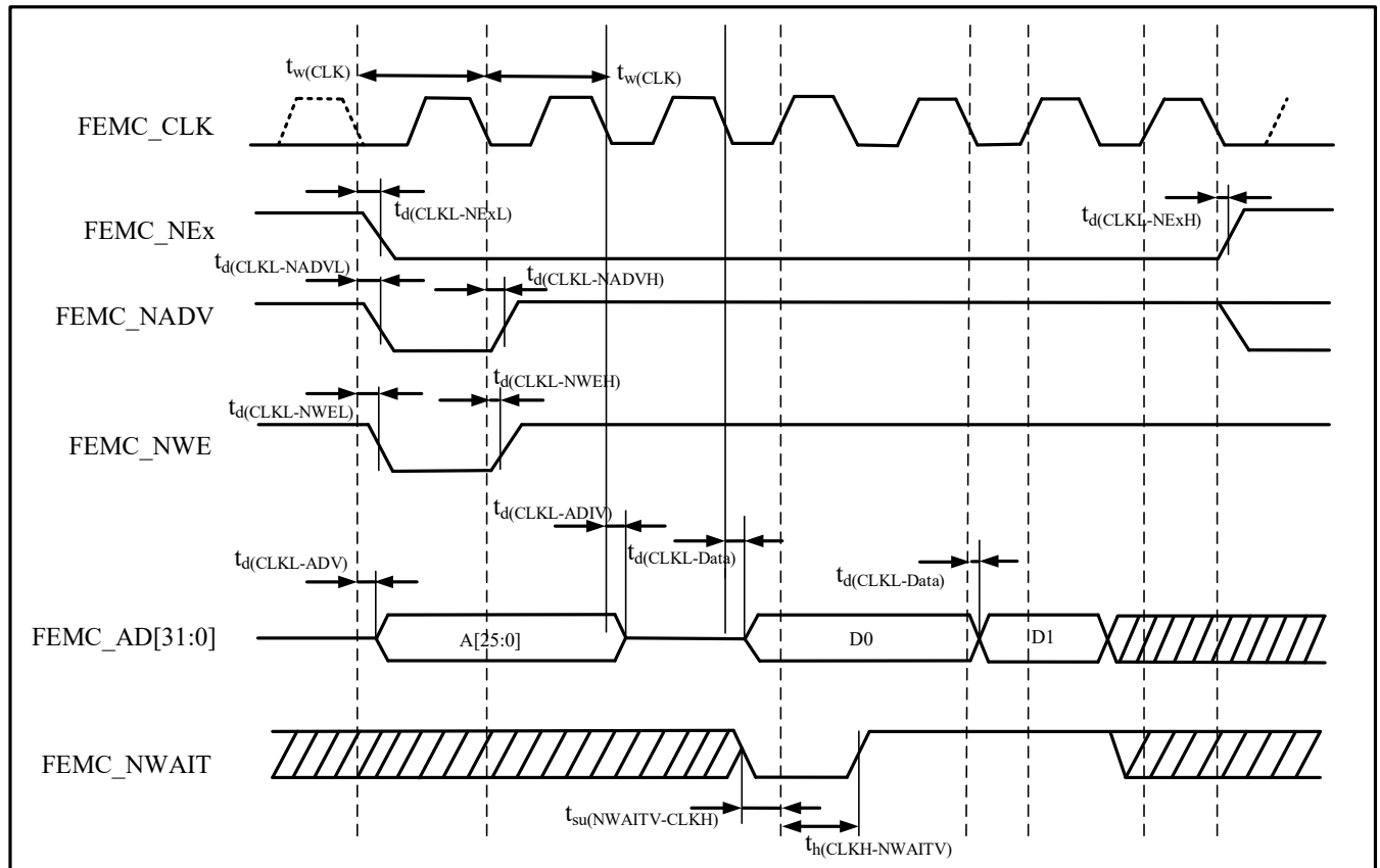
图 4-32 同步复用 PSRAM 写时序
