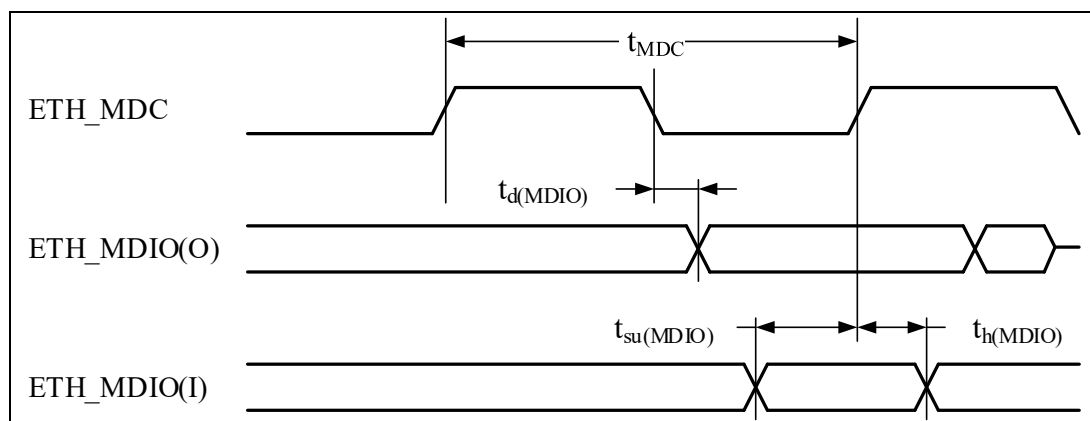
图 4-38 MDIO/SMA 时序图
