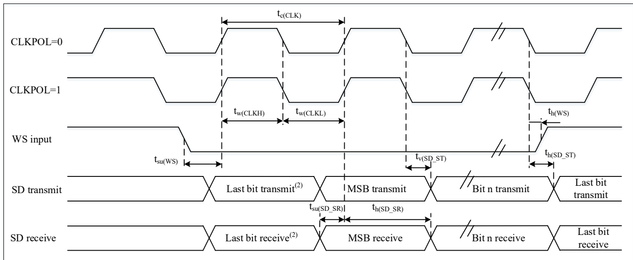
图 4-18 I 2 S 从模式时序图（飞利浦协议） (1)
