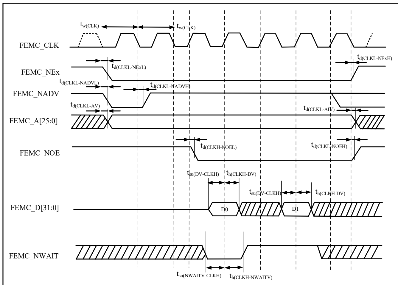
图 4-29 同步非总线复用 NOR/PSRAM 读时序
