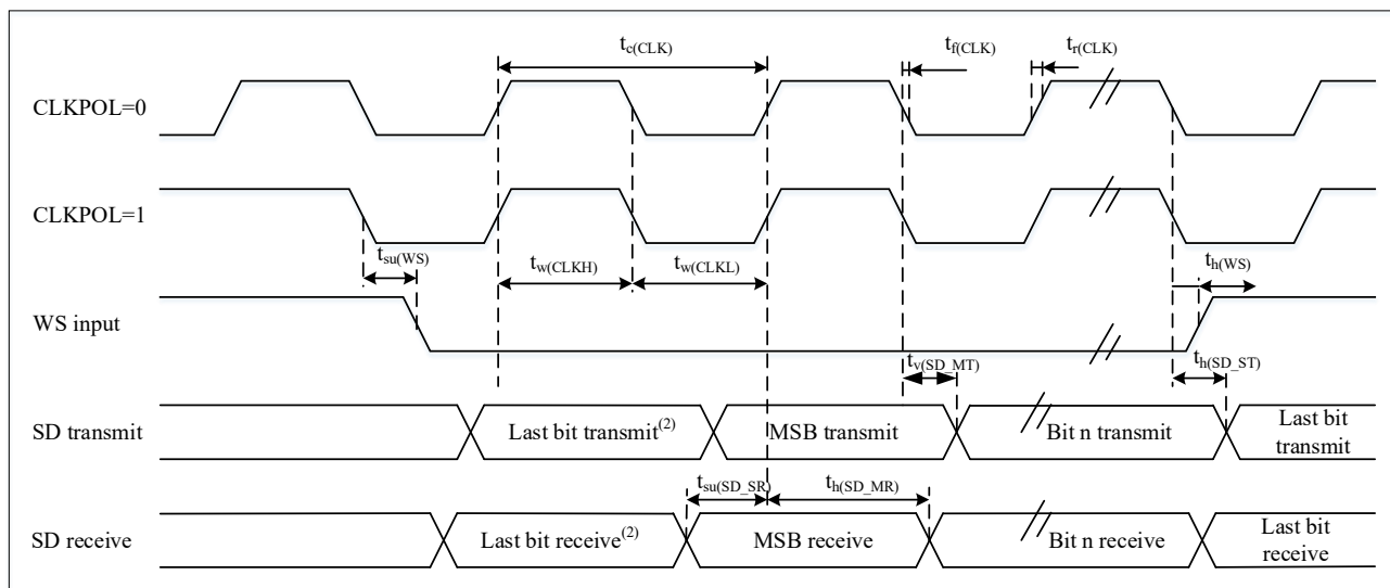
图 4-19 I 2 S 主模式时序图（飞利浦协议） (1)
