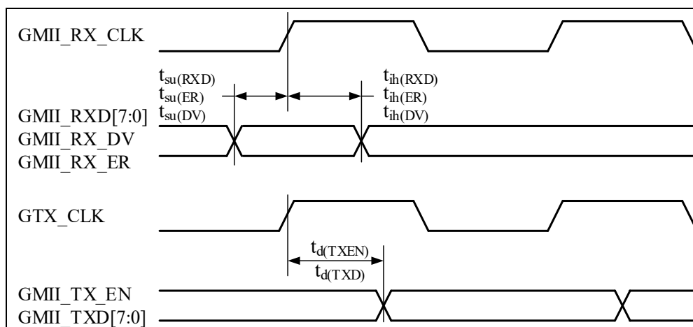
图 4-40 MII 时序图
