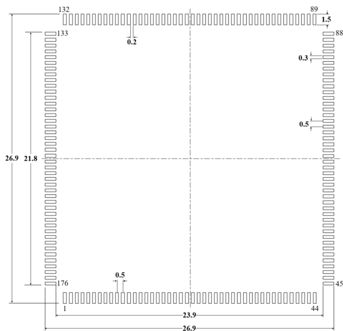
图 5-2 LQFP176 封装焊盘建议 (1)
