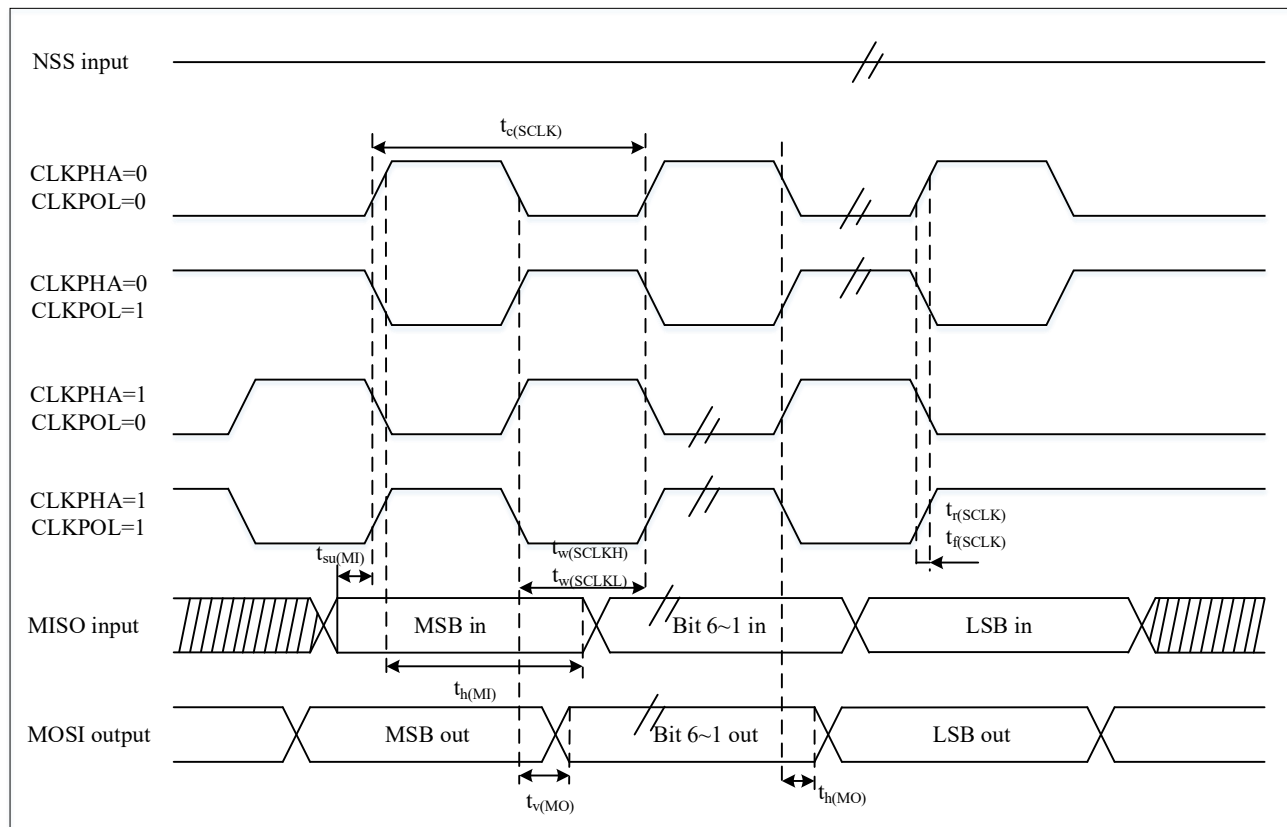
图 4-17 SPI 时序图 — 主模式 (1)
