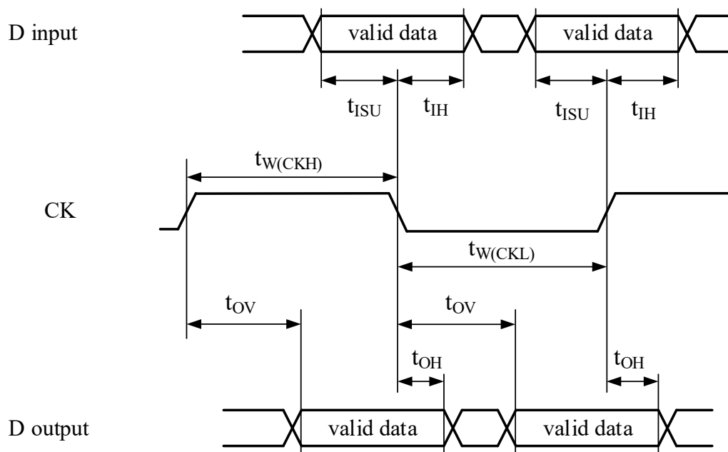
图 4-37 SDMMC DDR 模式
