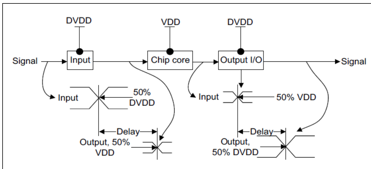
图 4-12 传输延迟
