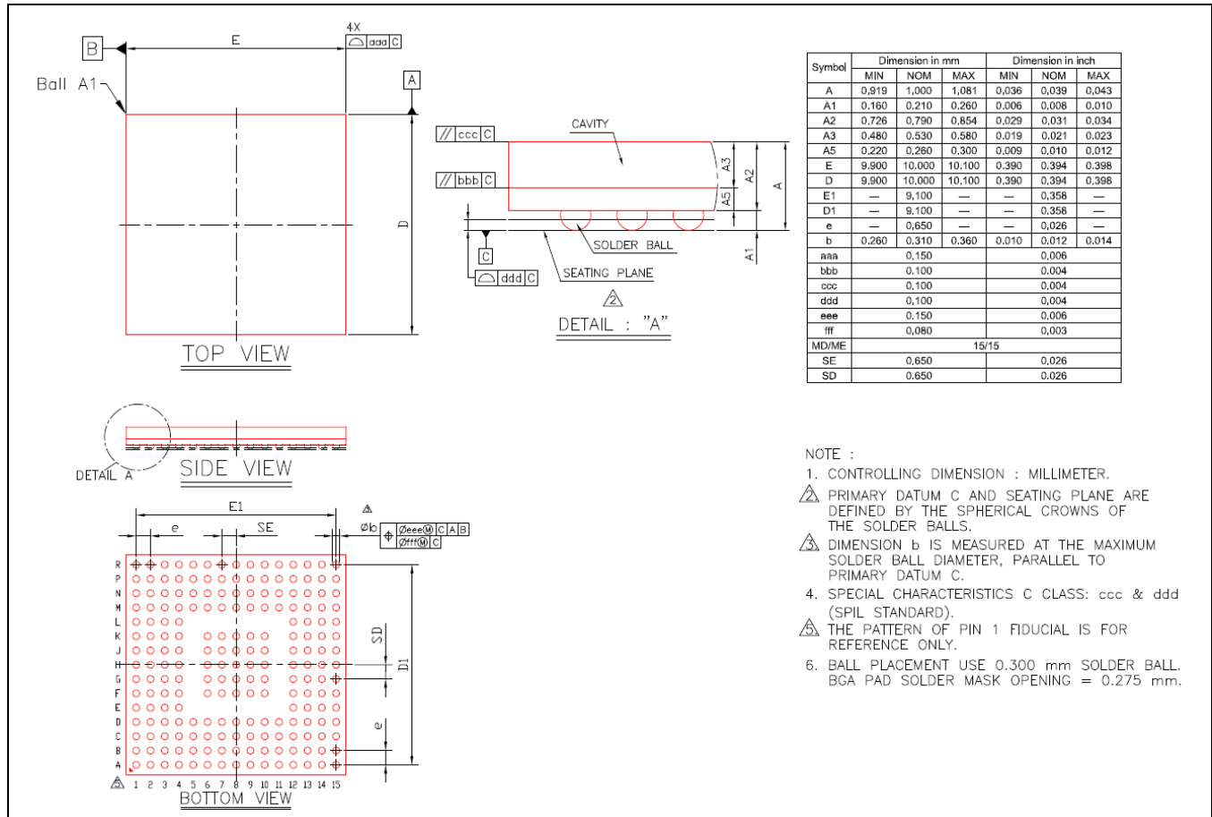
图 5-4 BGA176+25 封装焊盘建议
