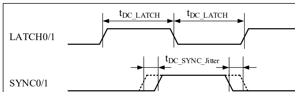
图 4-44 ESC Sync/Latch 信号时序图
