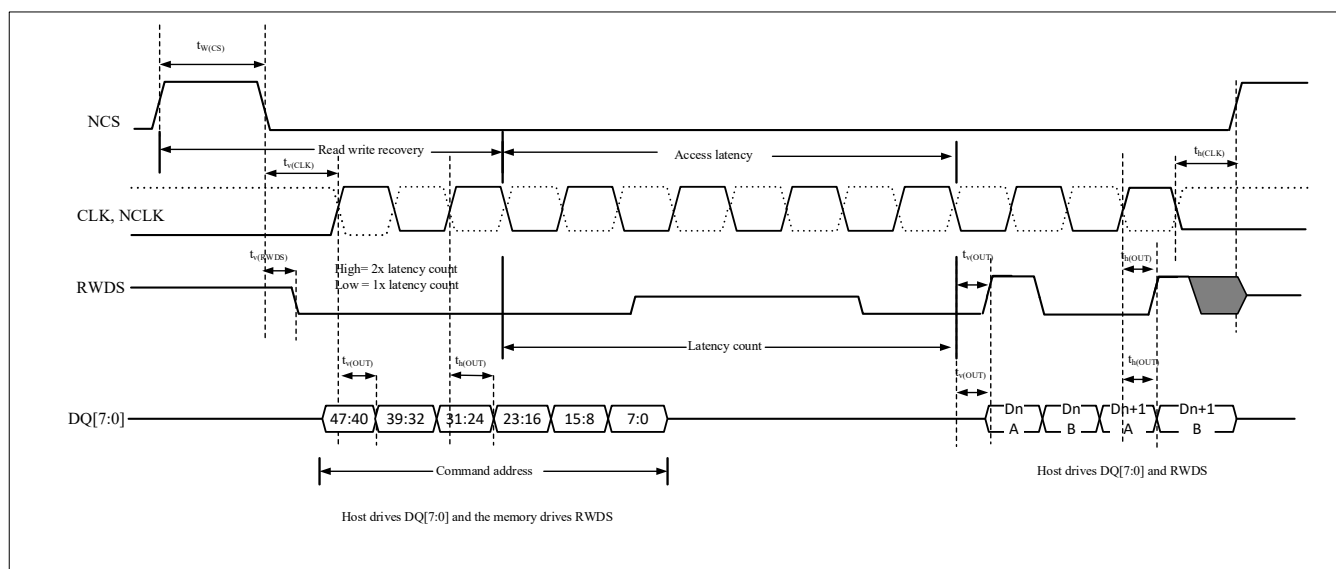
图 4-24 xSPI Hyperbus 时钟写时序图
