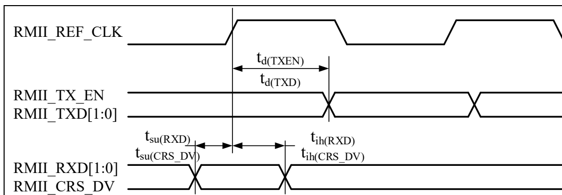
图 4-39 RMII 时序图
