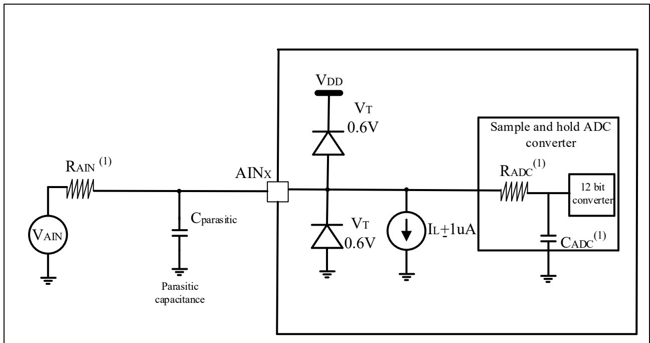
图 4-46 使用 ADC 典型的连接图
