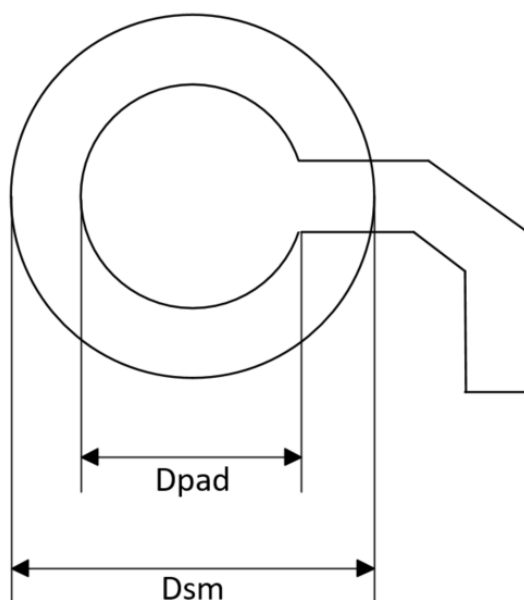
图 5-6 BGA176+25 封装焊盘建议
