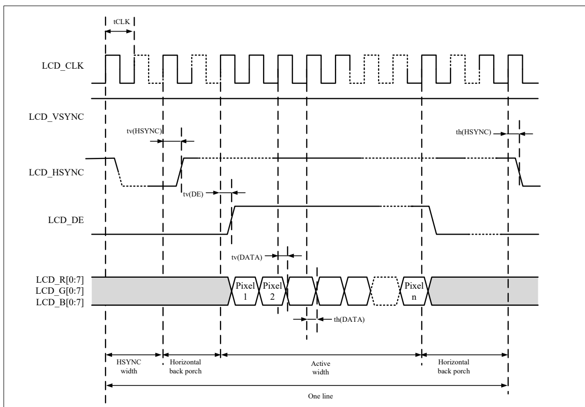
图 4-42 LCDC 水平时序框图
