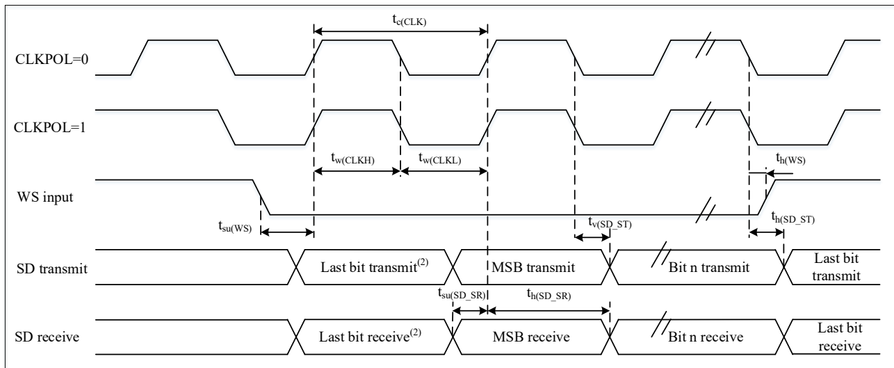
图 4-18 I 2 S 从模式时序图（飞利浦协议） (1)
