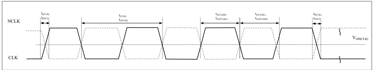
图 4-23 xSPI Hyperbus 时钟读时序图
