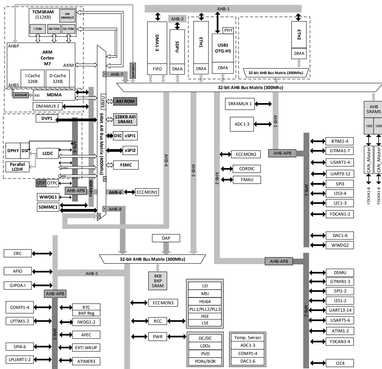
图 1-1 N32H735 系列框图
