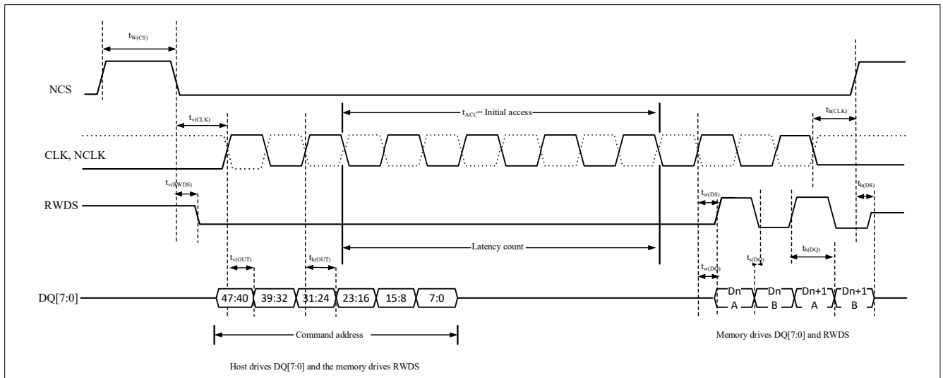
图 4-23 xSPI Hyperbus 时钟读时序图
