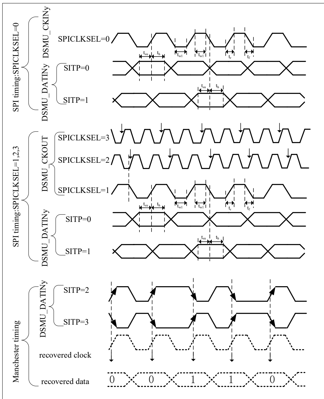
图 4-44 DSMU 通道收发器时序图
