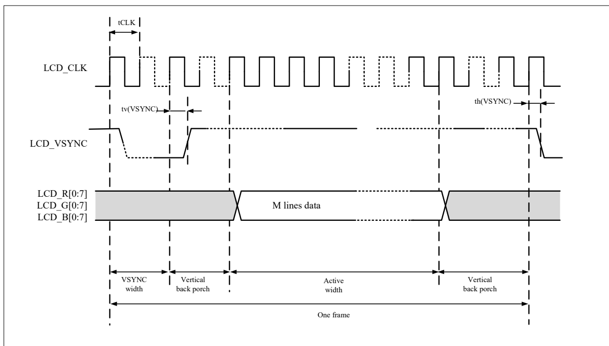
图 4-43 LCDC 垂直时序框图
