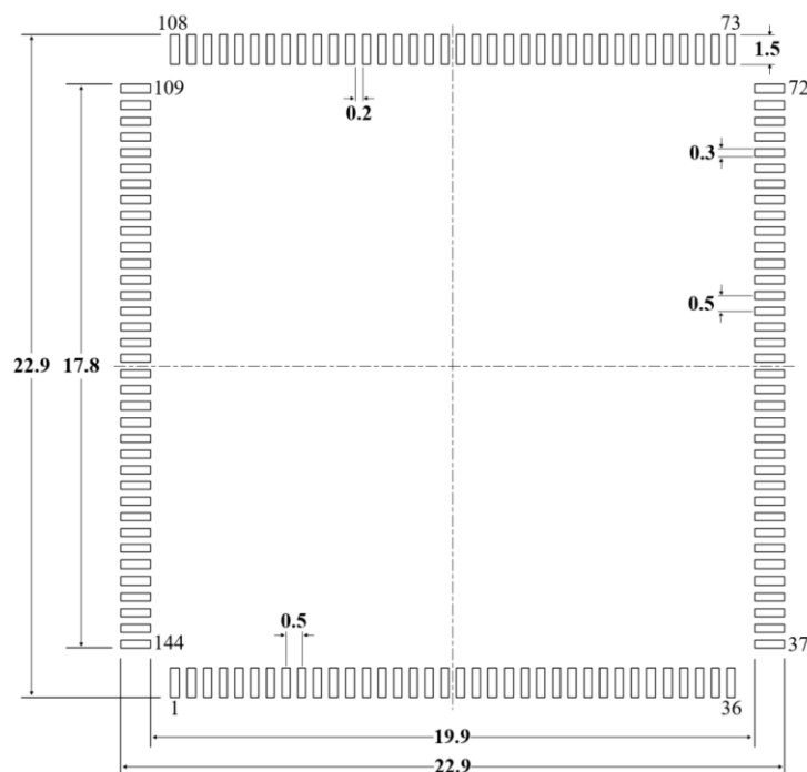
图 5-2 LQFP144 封装焊盘尺寸 (1)
