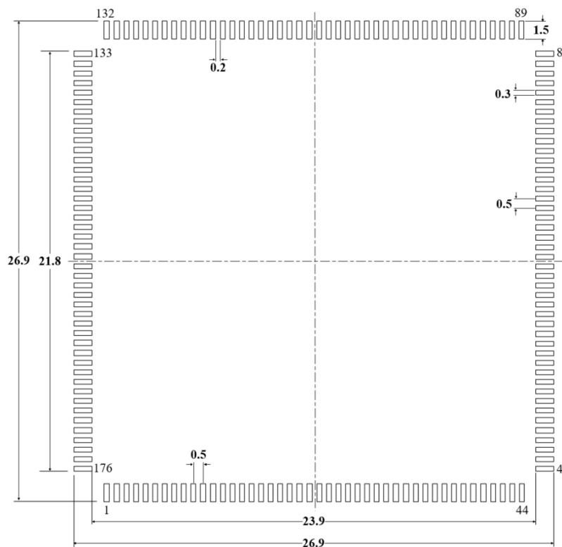
图 5-4 LQFP176 封装焊盘建议 (1)
